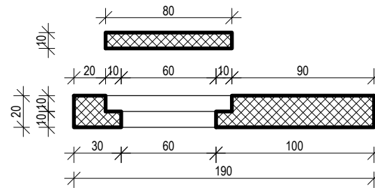
Gornja ploča s poklopcem presjek b-b
